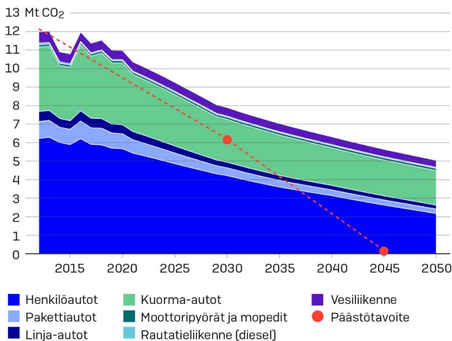
Kotimaan liikenteen CO 2 -päästöt, miljoonaa tonnia, perusennuste
